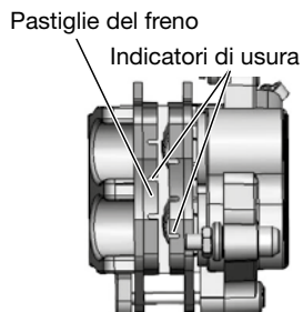
Freno anteriore
