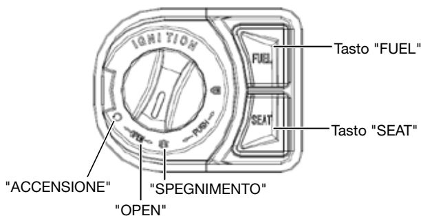
Blocchetto multifunzione
